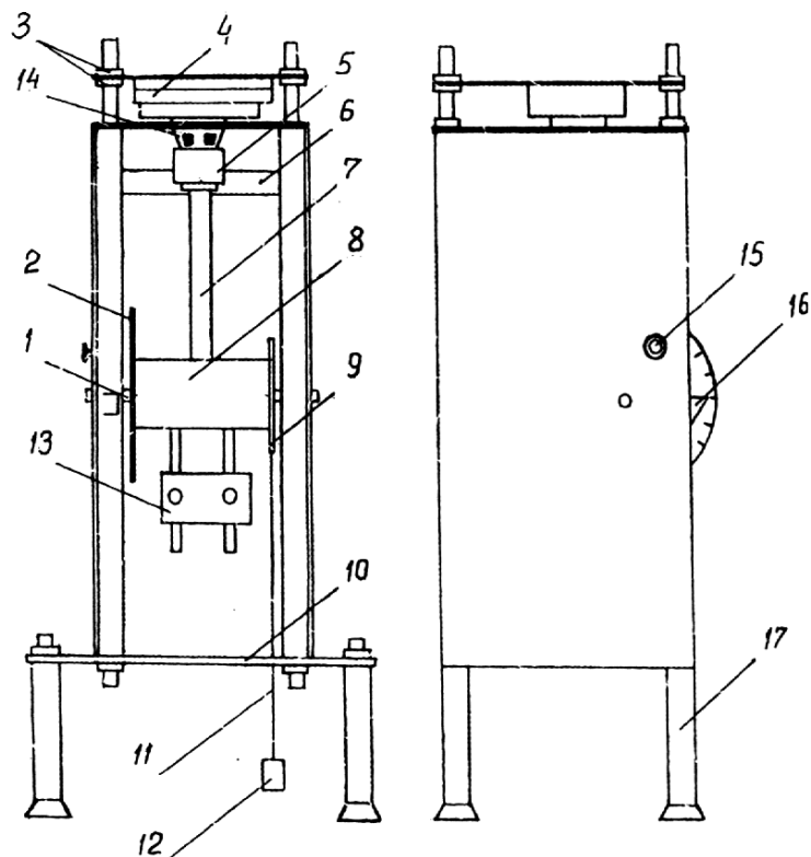
Схема стенда "ПРЯМОЙ УДАР":
